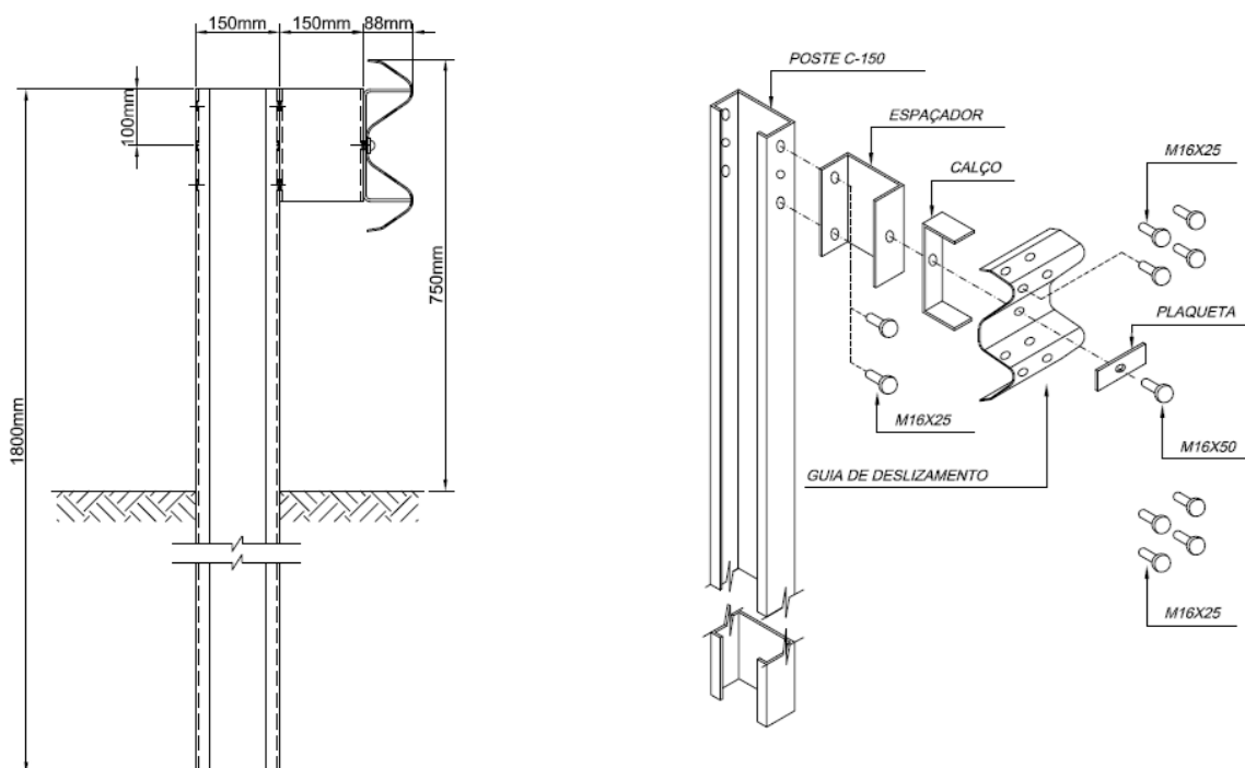
Detalhamento – Sistema de Defesa Metálica
