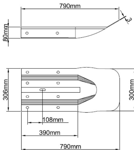
Detalhamento – Terminal – Ponteira Aérea
